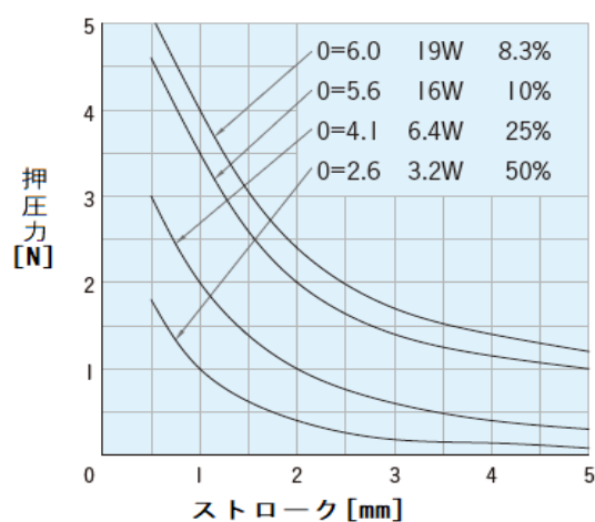
押圧力特性
