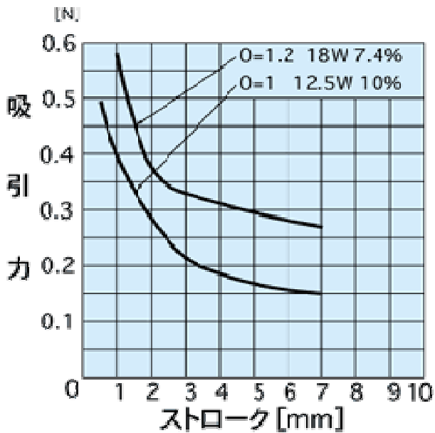
吸引力特性
