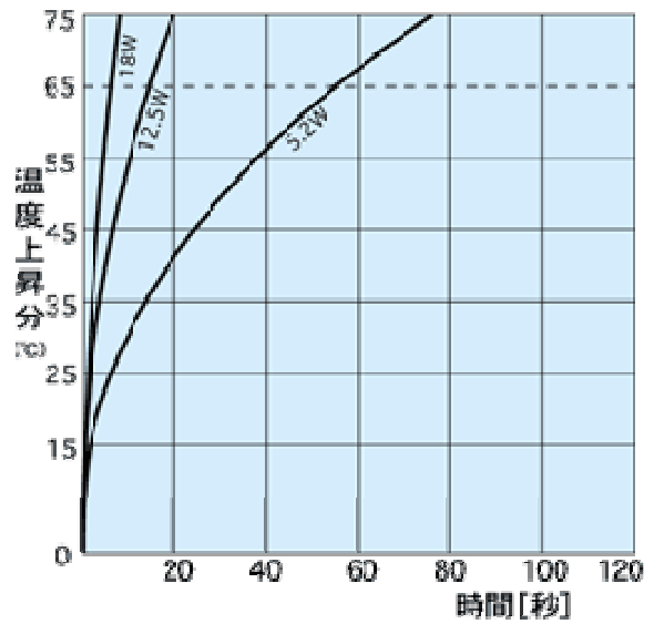
温度上昇特性
