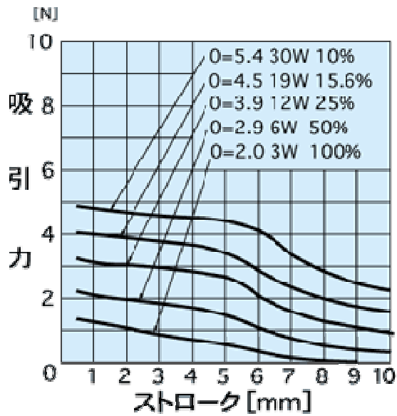
吸引力特性
